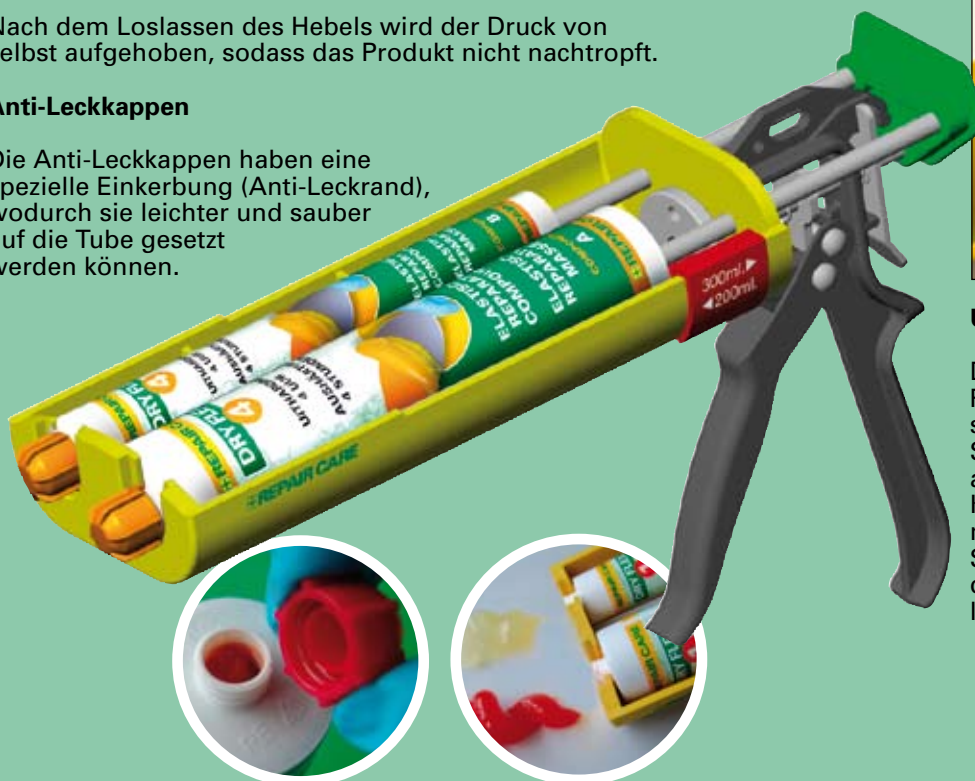
Anti-Leckkappen
